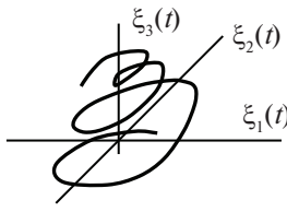
Векторные процессы (двумерный и трехмерный)
