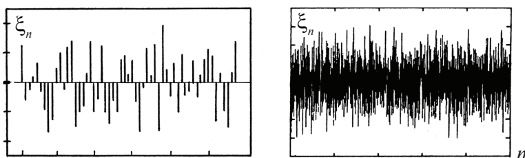
Реализации двух различных случайных последовательностей со статистически независимыми значениями
