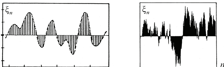
Случайные последовательности в данной ситуации порождены или управляются медленно изменяющимися процессами, и отдельные значения \xi_n не могут считаться здесь независимыми
