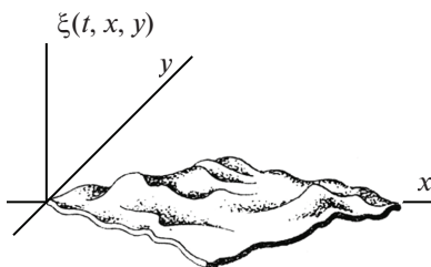
Реализация непрерывного пространственно-временного случайного поля
