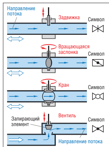
Рис. I.33. Виды арматуры
