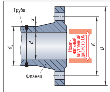
Рис. 1.3. Размеры труб
