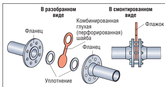
Рис. I.49. Комбинированный вариант глухой и перфорированной шайбы
