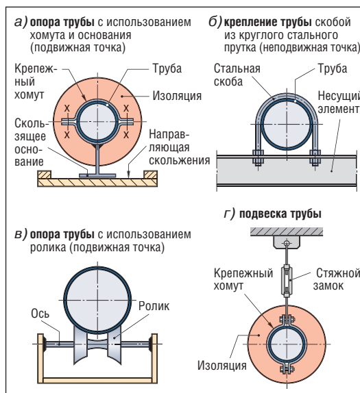
Рис. I.18. Крепления труб
