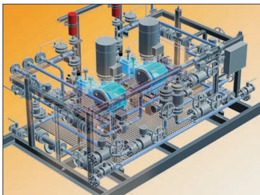
Рис. 1.31. Трехмерная CAD-модель установки
