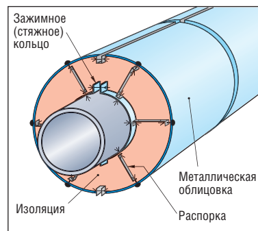
Рис. I.24. Изоляция трубы с использованием нижнего каркаса
