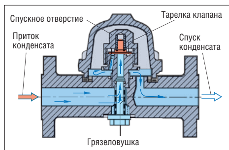
Рис. I.66. Термодинамический конденсатоотводчик
