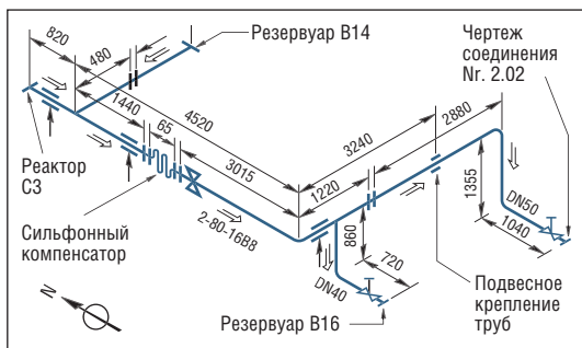
Рис. 1.30. Изометрическое изображение трубопровода
