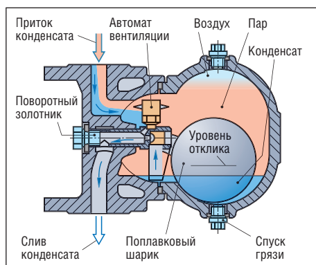
Рис. I.63. Поплавковый конденсатоотводчик
