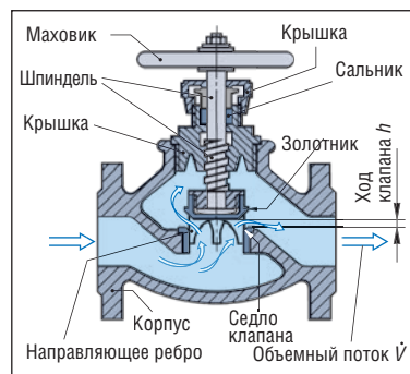
Рис. I.38. Конический вентиль (открыт)
