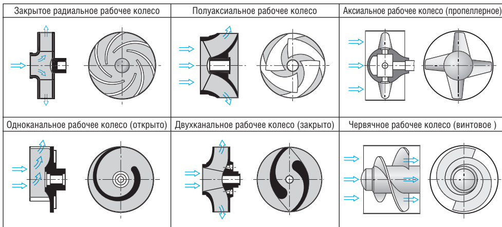
Рис. I.88. Формы рабочих колес у центробежных насосов (показан вид по оси сверху без крышки)
