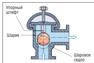
Рис. I.53. Шаровой клапан
