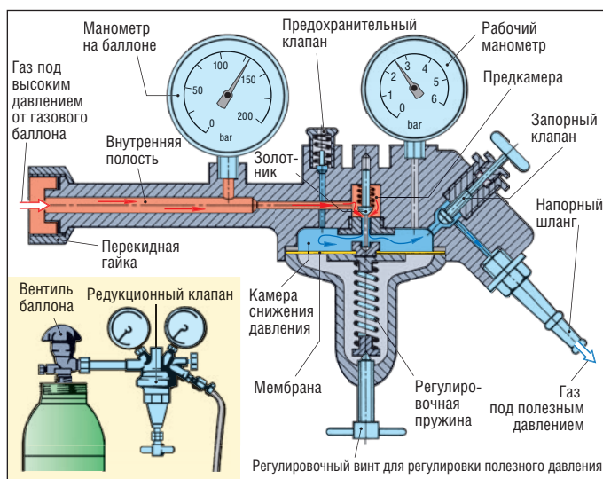
Рис. I.61. Редукционный клапан для газовых баллонов
