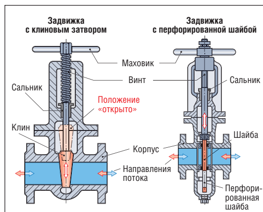
Рис. I.34. Конструктивные исполнения задвижек
