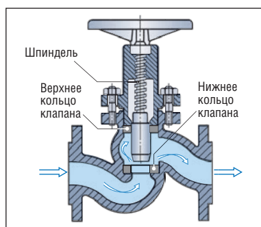
Рис. I.40. Цилиндрический вентиль (открыт)
