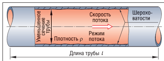
Рис. I.75. Факторы, влияющие на потерю давления
