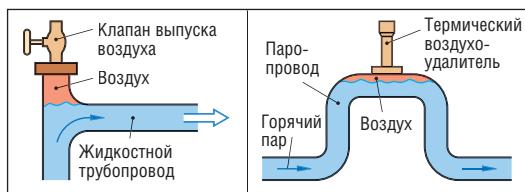
Рис. I.68. Порядок удаления воздуха
