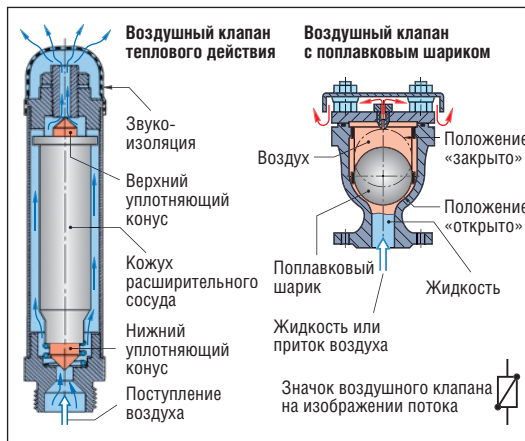
Рис. I.69. Конструктивные исполнения воздушных клапанов
