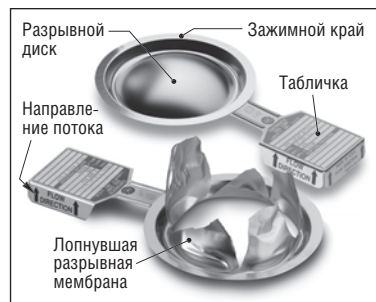
Рис. I.57. Разрывная мембрана
