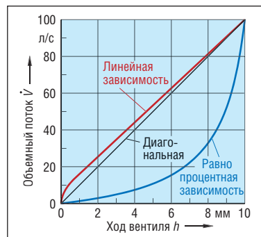
Рис. I.37. Характеристические линии вентиля
