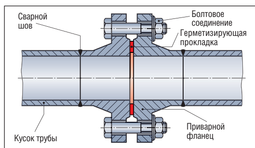
Рис. I.8. Фланцевое соединение
