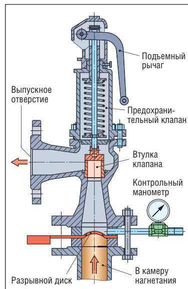
Рис. I.59. Предохранительный клапан со встроенными до него предохранителем с разрывной мембраной и устройством контроля давления
