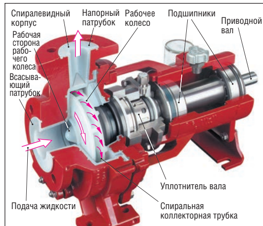
Рис. I.85. Взгляд внутрь центробежного насоса
