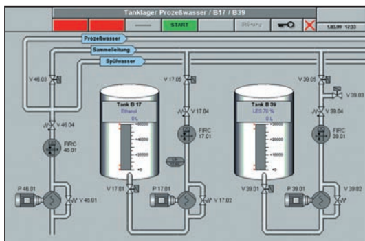
Рис. 1.29. Двумерная модель трубопроводов и устройств смесительной установки
