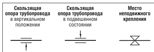
Рис. I.17. Условные обозначения креплений труб
