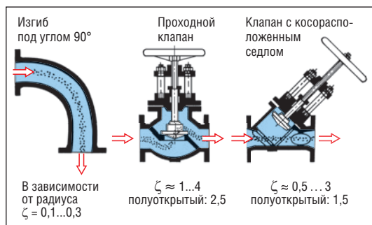
Рис. I.77. Коэффициенты местных сопротивлений
