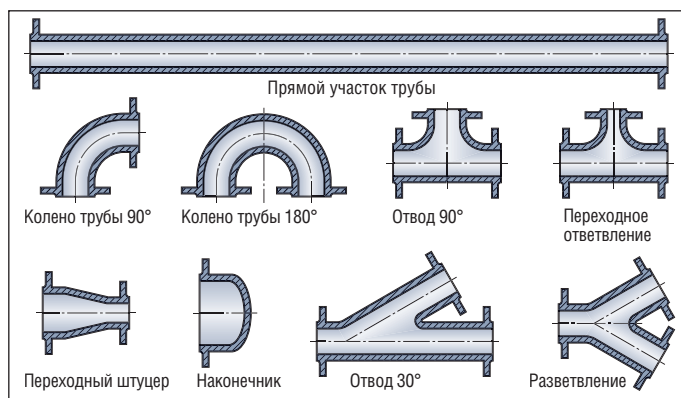
Рис. I.6. Фасонные части труб для сварки
