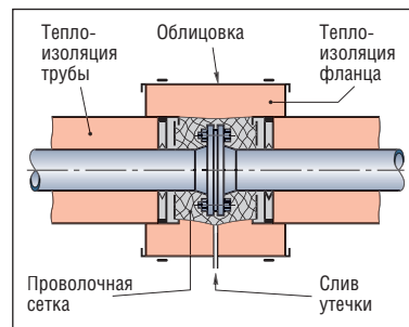
Рис. I.25. Теплоизоляция фланцевого соединения
