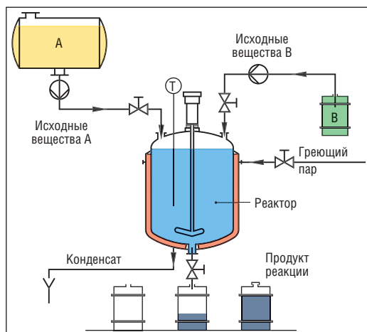
Рис. В.11. Химическая установка периодического действия
