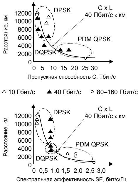
Рис. 2.18. Модуляционные форматы линий, в которых была достигнута производительность C \times L \approx 40 \text{ Пбит/с} \times \text{км} при емкости линии C > 1 \text{ Тбит/с}
