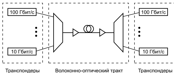
Рис. DWDM-система, общий вид
