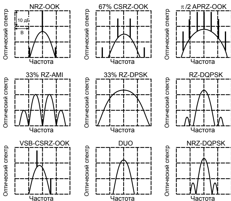
Рис. 2.19. Оптические спектры сигналов в различных форматах модуляции
