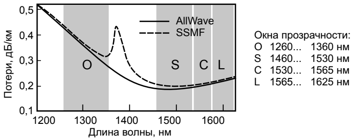
Рис. 2.2. Зависимость потерь в одномодовых волнах от длины волны света (SSMF — стандартное одномодовое волокно, AllWave — одномодовое волокно без «водяного пика»)
