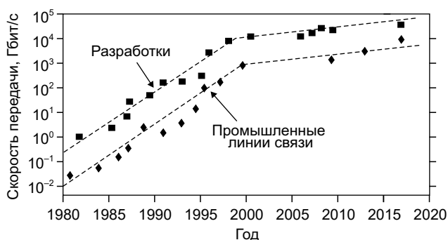
Рис. 1.2. Увеличение емкости лабораторных и промышленных линий связи начиная с 1980 г. После 2001 г. темп роста емкости линий уменьшился
