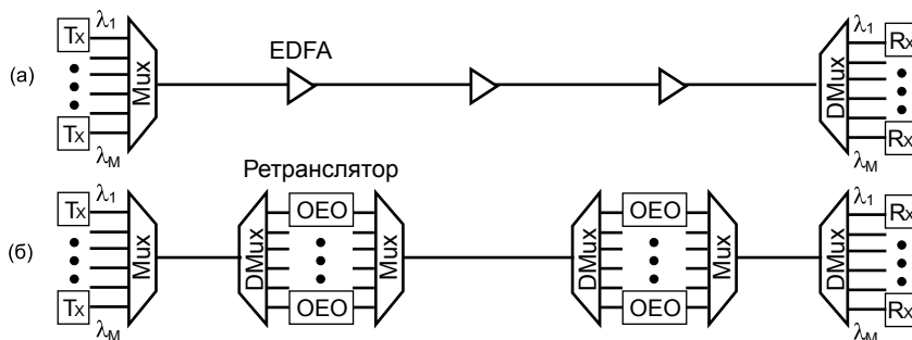
Рис. 2.4. Системы DWDM (а) с оптическими усилителями и (б) с OEO-регенераторами
