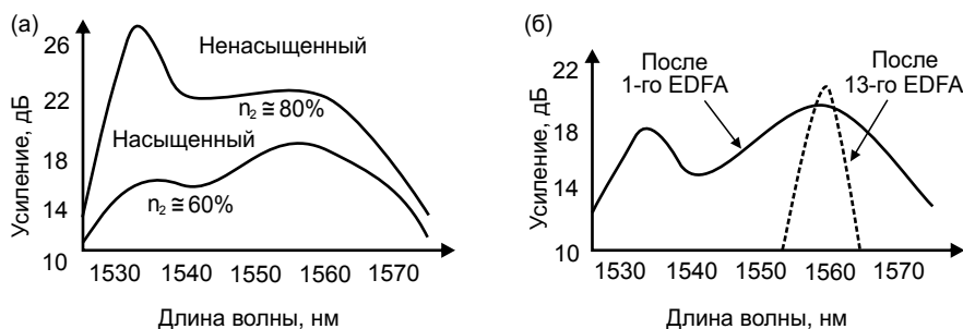
Рис. 2.11. Спектры усиления EDFA в диапазоне C в зависимости: (а) от населенности лазерных уровней и (б) от количества усилителей в каскаде
