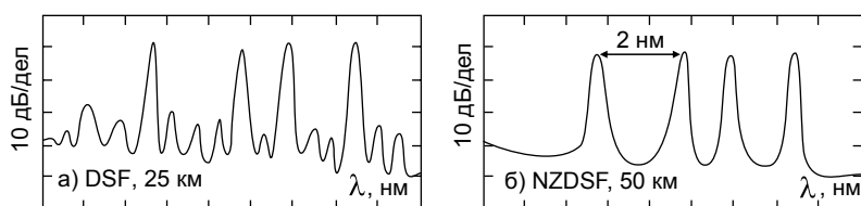
Рис. 2.8. Спектры сигналов на выходе DWDM-систем в С-диапазоне (мощность в канале ~3 дБм). (а) В DSF-волоках видны паразитные сигналы. (б) В NZDSF-волоках паразитных сигналов нет
