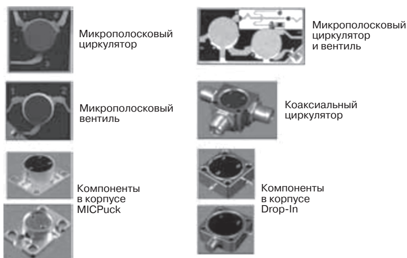
Рис. 11.8. Типы конструктивного исполнения вентиля, циркуляторов фирмы TRAK Microwave Ltd.
