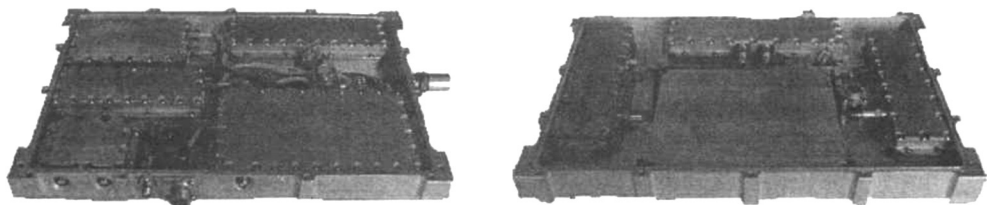
Рис. 11.41. Компоновка приемного и частотозадающего модуля 3-см диапазона
