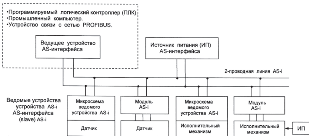
Рис. 1.14. Схема подключения устройств к AS-интерфейсу
