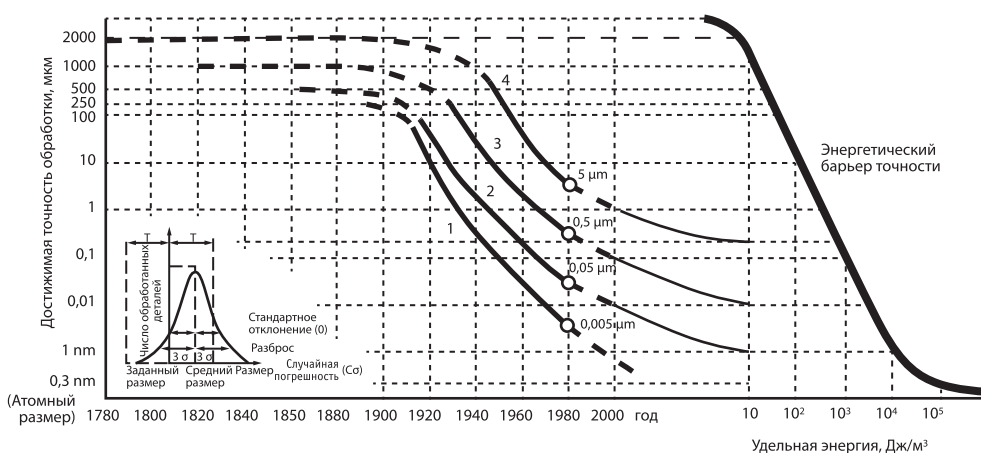
Рис. 1.8. Схема эволюции достижимой точности обработки. (1 — Сверхвысокоточная (ультрапрецизионная) обработка; 2 — Высокоточная (высокопрецизионная) обработка; 3 — Прецизионная обработка; 4 — Стандартная (нормальная) обработка)
