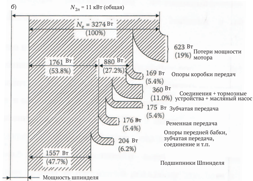
Рис. 1.17. Потери подводимой мощности при резании — а) [125]; потери в приводе станка — б) [120]
