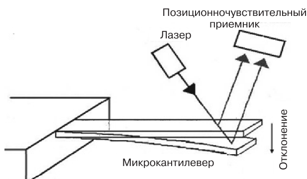
Рис. 1.8. Микрокантилевер с лазерным измерением величины смещения [63]
