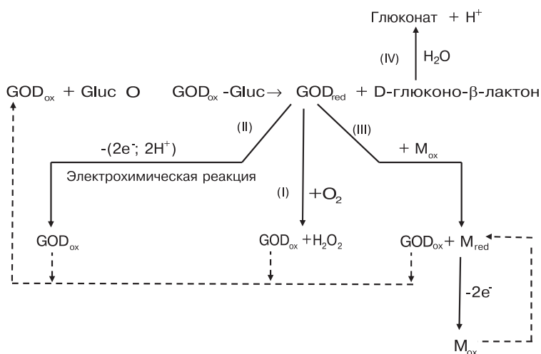
Рис. 3.12. Возможные методы преобразования для сенсоров на основе оксидазы глюкозы. GOD и Gluc обозначают оксидазу глюкозы и глюкозу соответственно
