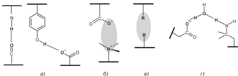
Рис. 2.8. Примеры нековалентных связей с включением боковых цепочек: а ) водородная связь; б ) ионная связь (соляной мостик); в ) гидрофобная связь ( R — гидрофобные боковые цепочки); г ) водяной мостик с водородной связью между карбоксильной и аминной группой. Толстые линии представляют собой основы протеина
