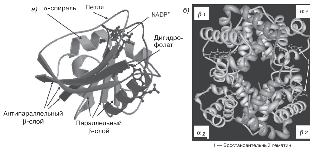
Рис. 2.7. а) Третичные структуры кишечной палочки фермента дигидрофолатредуктазы в качестве третичной структуры с основой (дигидрофолат) и коферментом \text{NADP}^+ . Взято из http://www.rcsb.org/pdb/explore/explore.do?structureId=1DRE . б) Четвертичная структура гемоглобина. Также показаны группы гемо-железа. Взято из http://www.rcsb.org/pdb/explore/explore.do?structureId=1A3N . Последний доступ: 15.05.2012
