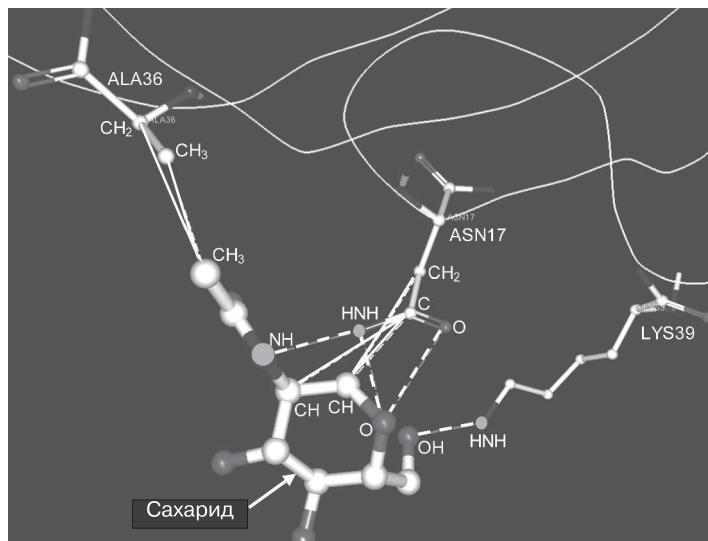
Рис. 2.10. Соединение сахара (2-(ацетиламино)-2-деокси- \alpha -D-глюкопираноза) с авидином. Сплошные прямые линии: гидрофобные связи; пунктирная линия: водородные связи. Взято из: http://www.rcsb.org/pdb/explore/explore.do?structureId=2AVI . Последний доступ: 15.05.2012
