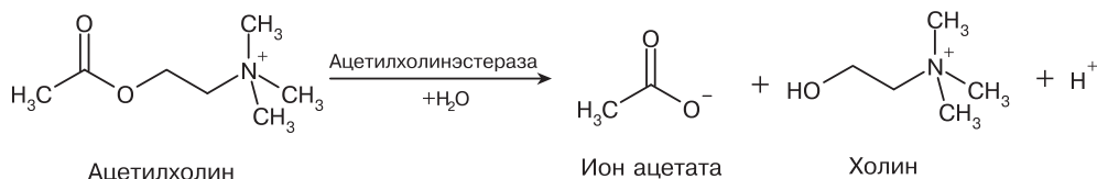
Рис. 3.10. Ферментативный гидролиз ацетилхолина
