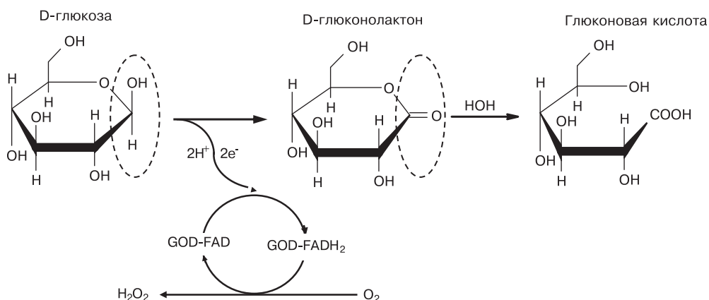
Рис. 3.9. Окисление глюкозы катализируется оксидазой глюкозы (GOD). Соответственно FAD и FADH 2 являются окисдованными и восстановленными формами простетической группы. Глюкоза окисляется посредством передачи электронов и ионов водорода окисленной форме простетической группы (FAD), которая восстанавливается до FADH 2 с молекулярным водородом. При этой реакции перекись водорода образуется как побочный продукт
