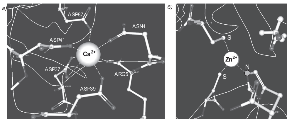
Рис. 2.9. Связь ионов металла в протеинах: а) ион кальция поддерживается электростатическими связями в кальдереине 23. Взято из http://www.rcsb.org/pdb/explore/explore.do?structureId=2WBX . б) \text{Zn}^{2+} в алкогольной дегидрогеназе. Координация металла выполняется двумя атомами серы из остатков цистеина и азотом из имидазольного кольца в остатке гистидина. Кривые линии отображают основу протеина. Взято из http://www.rcsb.org/pdb/explore/explore.do?structureId=1SBY . Последнее посещение: 15.05.2012
