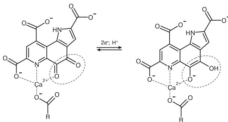
Рис. 3.7. Кофактор пирролохинолинхинон (PQQ). R обозначает остаток протеина
