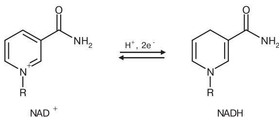
Рис. 3.6. Окислительно-восстановительная реакция амидадениндинуклеотида. Показанное реагирующее вещество — никотинамид; R обозначает остальную часть молекулы кофермента
