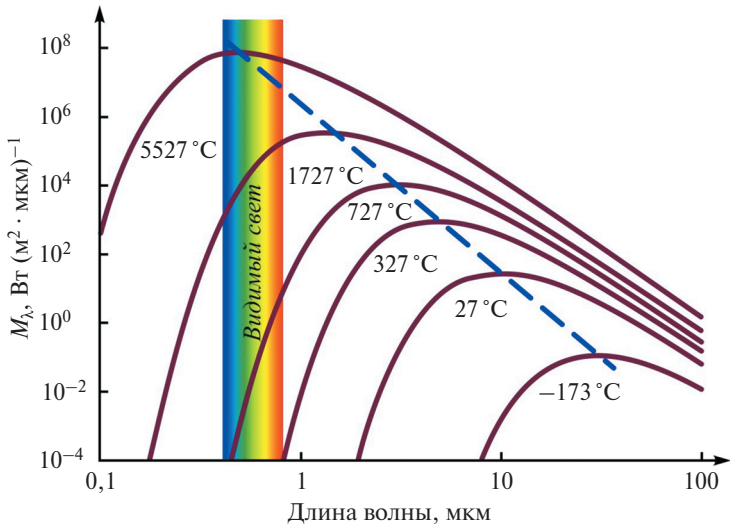
Рис. 1.1. Зависимость интенсивности излучения от длины волны для абсолютно черного тела при различной температуре в соответствии с законом Планка. Штриховая линия отвечает смещению максимума интенсивности при изменении температуры в соответствии с законом Вина [7]
