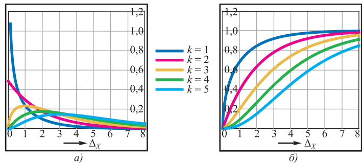
Рис. 1.6. Графики плотностей вероятностей (а) и функций распределения хи-квадрат (б)
