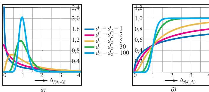
Рис. 1.8. Графики плотностей вероятности (а) и функций распределения Фишера (б)
