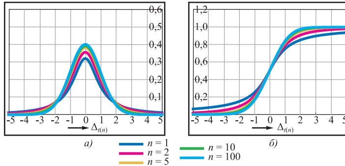
Рис. 1.7. Графики плотностей вероятностей (а) и функций распределения Стьюдента (б)
